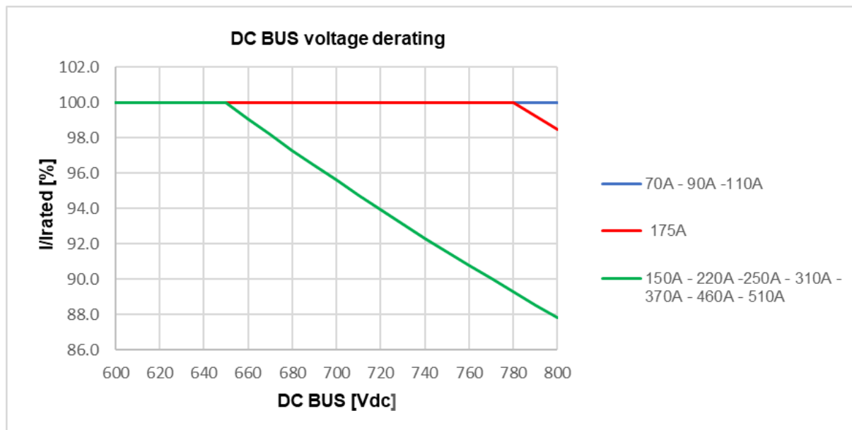
FIG. 9 - Declassamento tensione d'ingresso / Input voltage derating
