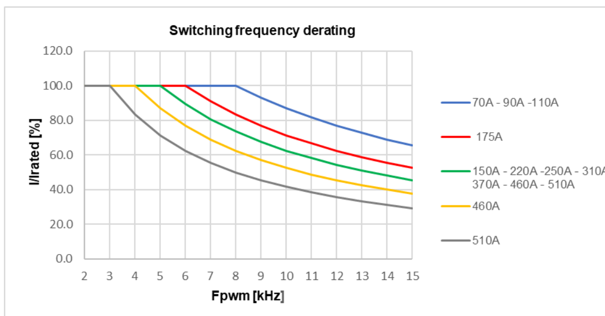
FIG. 12 - Declassamento frequenza di switching / Switching frequency derating
